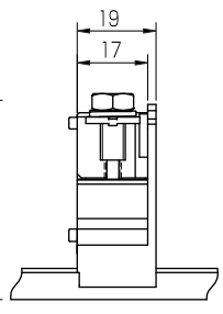
適合圧着端子
