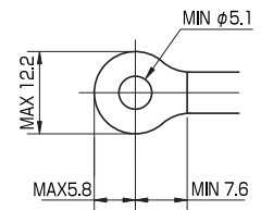
適合圧着端子
