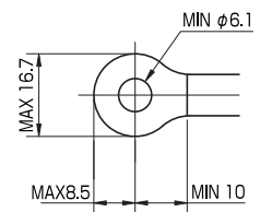
適合圧着端子
